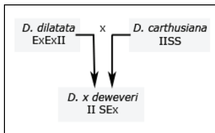
Fig. 7. Esquema de relaciones genómicas de Dryopteris dilatata , D. carthusiana y D. × deweveri . Ver texto.
