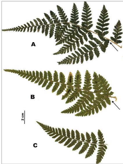
Fig. 6. Fotosiluetas: comparativa de las pinnas basales de A , Dryopteris dilatata (Cantabria: 30TVN38, Selaya pr. Pisueña, 320 m, 15-VI-2006); B , D. × deweveri (especimen nº 8); C , D. carthusiana (Cantabria: 30TVN38, Selaya pr. Pisueña, id).
